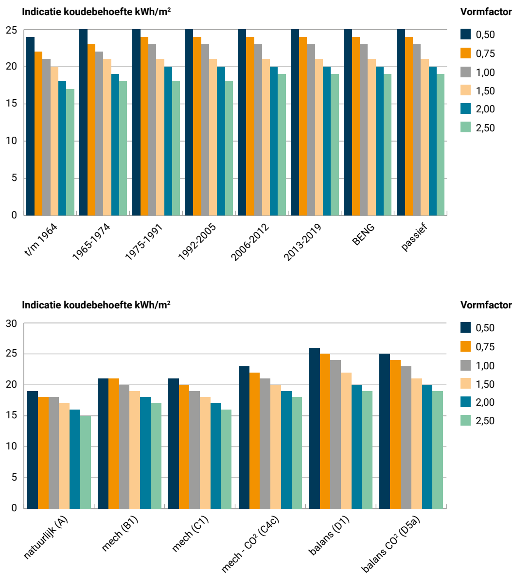
Figuur 3 Berekende koudebehoefte woningen bij verschillend woningtype, ventilatiesysteem en isolatiegraad
